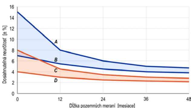
Obr. 4. Presnosť solárneho modelu vo vybranej lokalite alebo regióne je možné zvýšiť využitím kvalitných lokálnych dát
