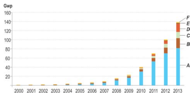
Obr. 8. Vývoj inštalovanej kapacity fotovoltických elek-
