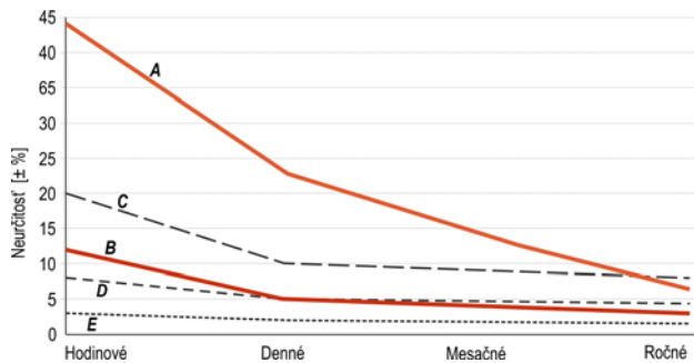
Obr. 2. Porovnanie presnosti modelu SolarGIS s kvalitnými dátami
