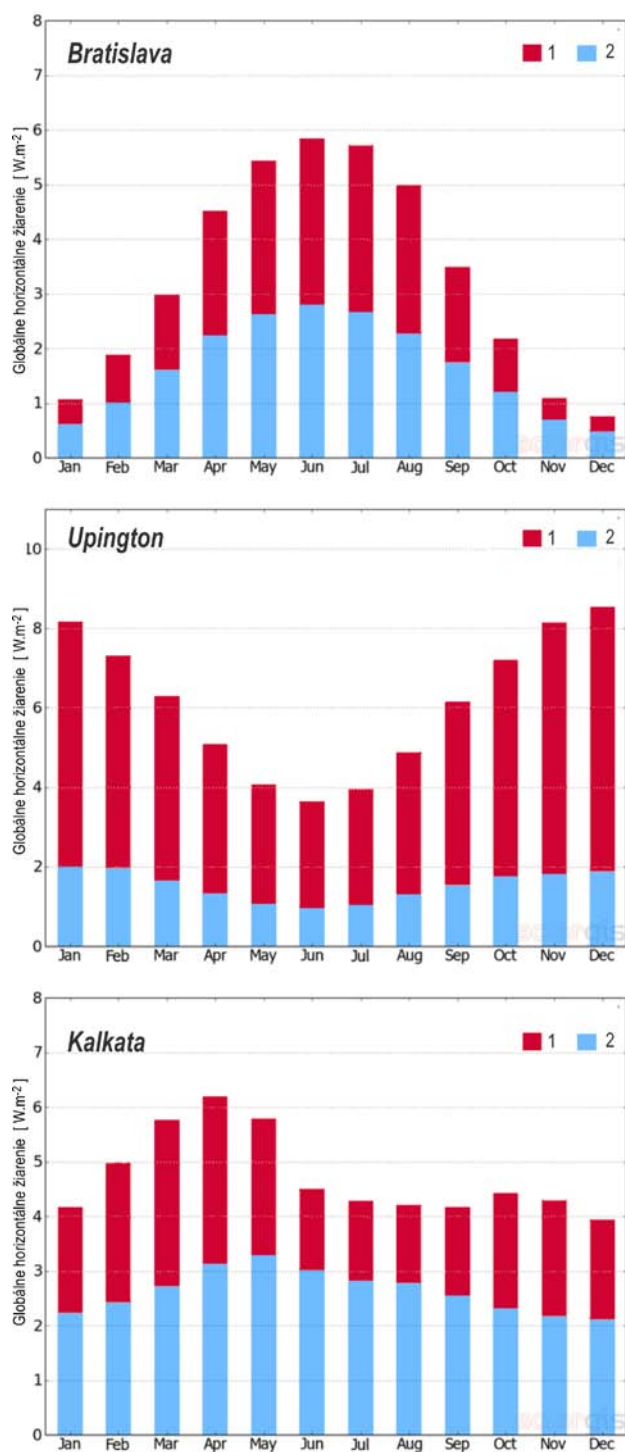
Obr. 6. Dlhodobé mesačné priemery globálneho horizontálneho
